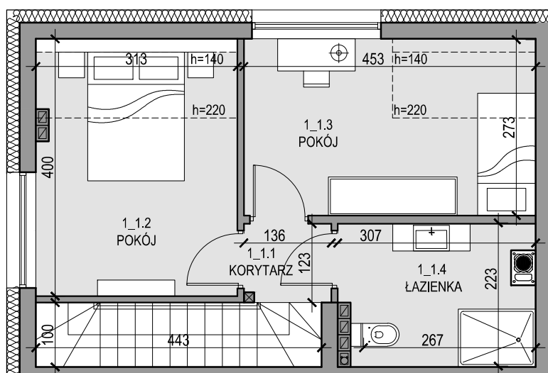
RZUT PIĘTRA
